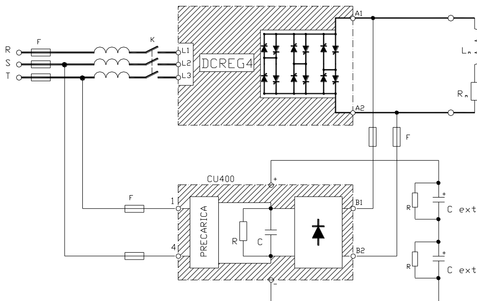
Figura 3: Collegamento condensatori
